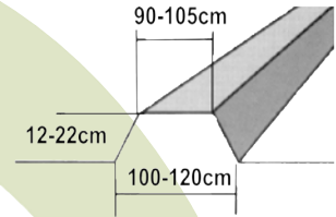
ΕΝΔΕΙΚΤΙΚΕΣ ΔΙΑΣΤΑΣΕΙΣ ΑΝΑΧΩΜΑΤΟΣ
