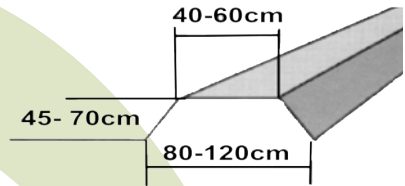
ΕΝΔΕΙΚΤΙΚΕΣ ΔΙΑΣΤΑΣΕΙΣ ΑΝΑΧΩΜΑΤΟΣ
