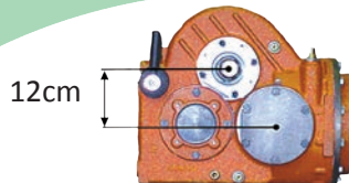
ΣΑΣΜΑΝ COMER, ΜΕ ΤΥΠΟ ΜΖ-3Α
