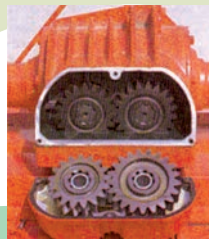
ΣΑΣΜΑΝ COMER, ΜΕ ΤΥΠΟ MZ-3A
