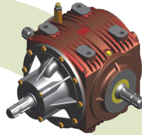
ΚΕΝΤΡΙΚΟΣ ΜΕΙΩΤΗΡΑΣ COMER ΤΥΠΟΥ T-331
