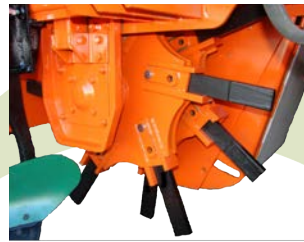
ΣΤΡΟΦΕΙΟ ΠΑΤΕΝΤΑΡΙΣΜΕΝΟ ΜΕ ΥΠΟΔΟΧΕΣ ΓΙΑ ΜΑΧΑΙΡΙΑ ΚΑΙ ΣΤΗΡΙΞΗ ΜΕ ΠΕΙΡΟ ΜΕ ΔΥΝΑΤΟΤΗΤΑ ΜΕΤΑΤΟΠΙΣΗΣ 3 ΦΟΡΕΣ
