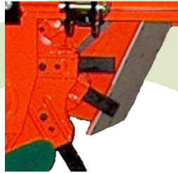
ΣΤΡΟΦΕΙΟ ΠΑΤΕΝΤΑΡΙΣΜΕΝΟ ΜΕ ΥΠΟΔΟΧΕΣ ΓΙΑ ΜΑΧΑΙΡΙΑ ΚΑΙ ΣΤΗΡΙΞΗ ΜΕ ΠΕΙΡΟ ΜΕ ΔΥΝΑΤΟΤΗΤΑ ΜΕΤΑΤΟΠΙΣΗΣ 3 ΦΟΡΕΣ
