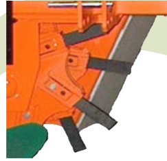
ΣΤΡΟΦΕΙΟ ΠΑΤΕΝΤΑΡΙΣΜΕΝΟ ΜΕ ΥΠΟΔΟΧΕΣ ΓΙΑ ΜΑΧΑΙΡΙΑ ΚΑΙ ΣΤΗΡΙΞΗ ΜΕ ΠΕΙΡΟ ΜΕ ΔΥΝΑΤΟΤΗΤΑ ΜΕΤΑΤΟΠΙΣΗΣ 3 ΦΟΡΕΣ
