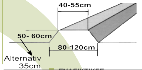
ΕΝΔΕΙΚΤΙΚΕΣ ΔΙΑΣΤΑΣΕΙΣ ΑΝΑΧΩΜΑΤΟΣ
