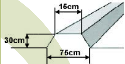
ΕΝΔΕΙΚΤΙΚΕΣ ΔΙΑΣΤΑΣΕΙΣ ΑΝΑΧΩΜΑΤΟΣ
