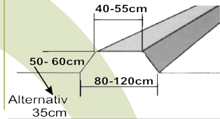
ΕΝΔΕΙΚΤΙΚΕΣ ΔΙΑΣΤΑΣΕΙΣ ΑΝΑΧΩΜΑΤΟΣ
