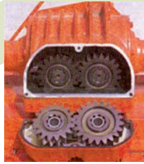
ΣΑΣΜΑΝ COMER, ΜΕ ΤΥΠΟ ΜΖ-3Α
