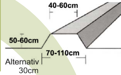
ΕΝΔΕΙΚΤΙΚΕΣ ΔΙΑΣΤΑΣΕΙΣ ΑΝΑΧΩΜΑΤΟΣ
